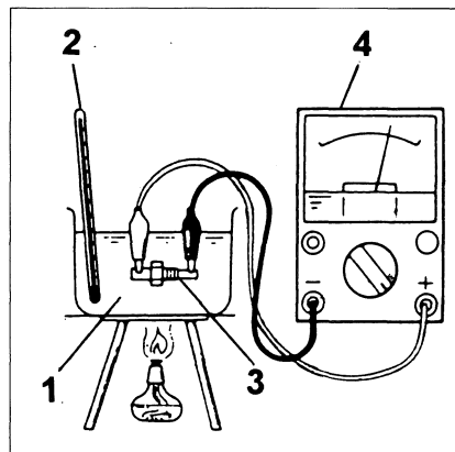
Contrôle de la résistance de l'électrovanne à l'aide d'un ohmmètre.
