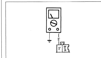
Contrôle du contacteur de point mort.
