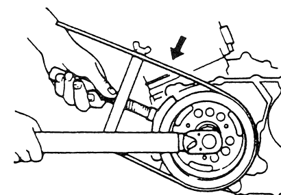
Méthode d'immobilisation d'un rotor d'alternateur avec l'outil Yamaha (réf. 90080-01701)
