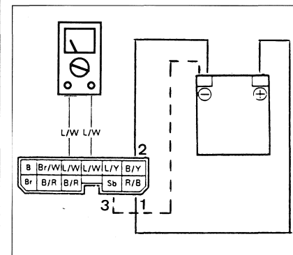
Contrôle du relais de coupure de démarrage à l'aide d'un Ohmmètre et d'une batterie branchée en 1 et 2 puis en 1 et 3.
