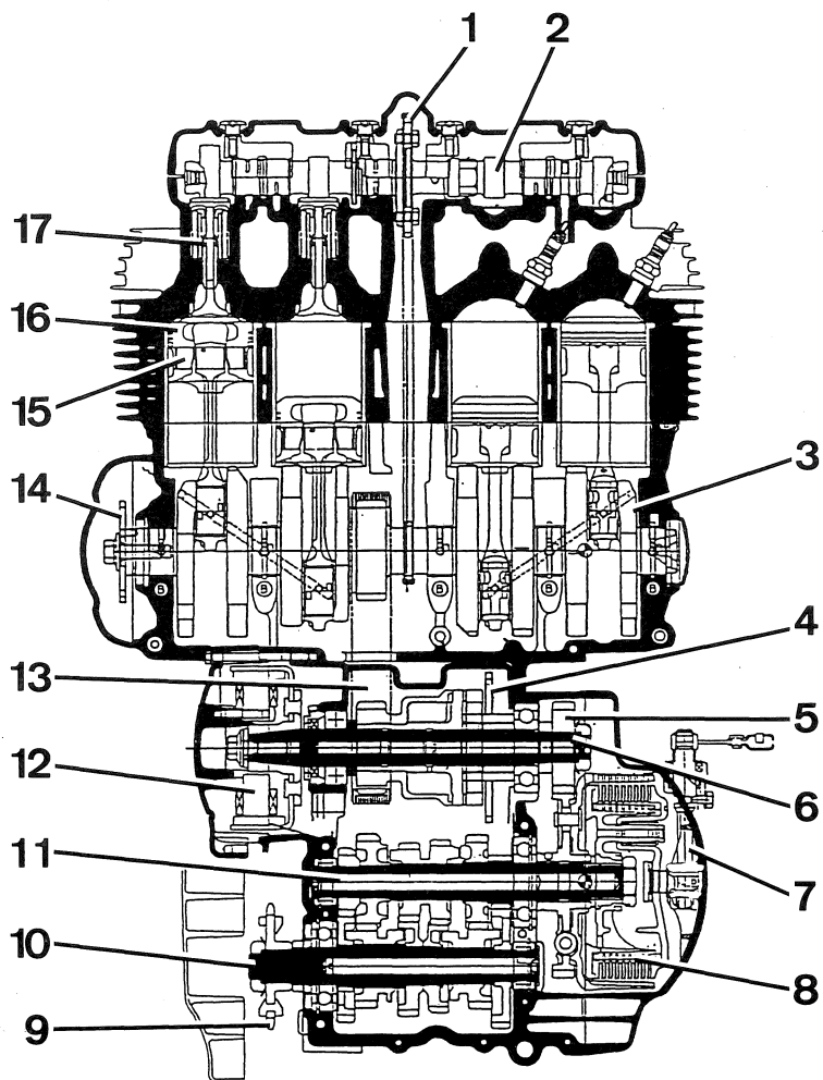
COUPE HORIZONTALE DU MOTEUR
