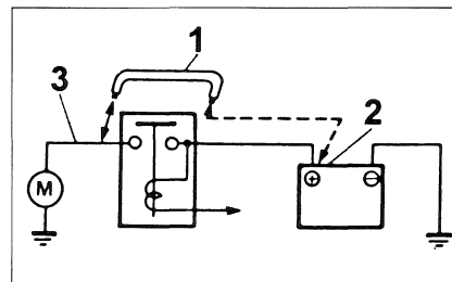
Contrôle du démarreur.
