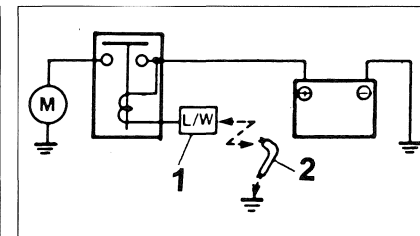
Contrôle du relais de démarreur.
