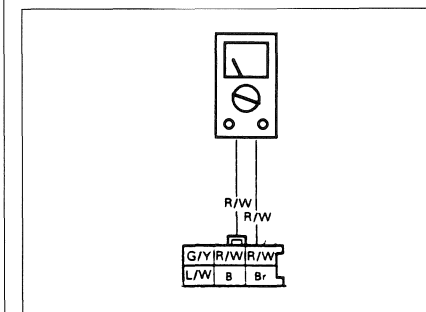
Contrôle du coupe-circuit de sécurité
