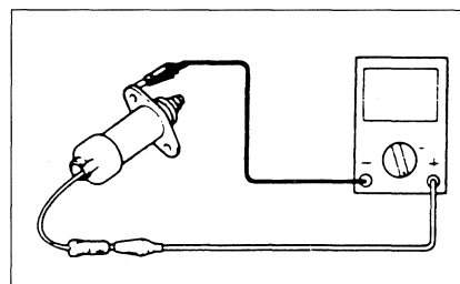
Contrôle de la résistance de l'électrovanne à l'aide d'un ohmmètre.
