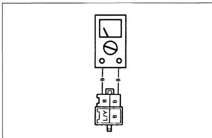
Contrôle du contacteur de béquille latérale.
