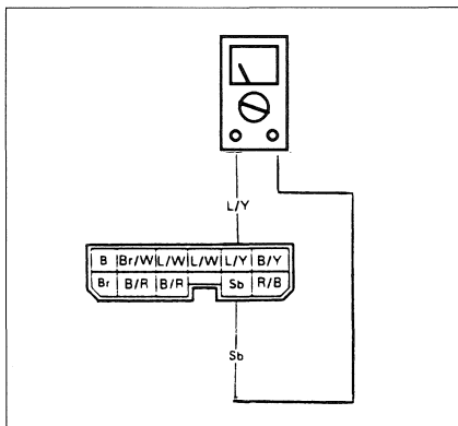
Contrôle de la diode du bloc relais.
