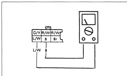
Contrôle du contacteur de démarrage
