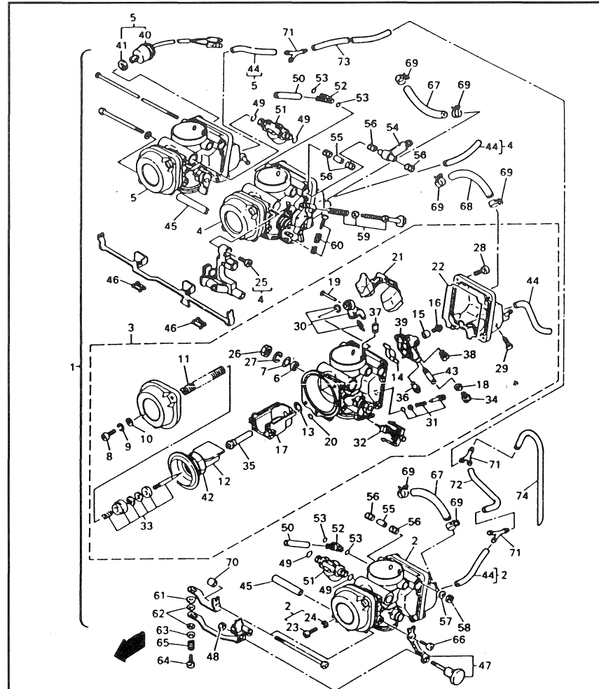
RAMPE DE CARBURATEURS
