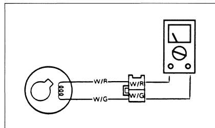
Contrôle de la résistance du capteur d'allumage.
