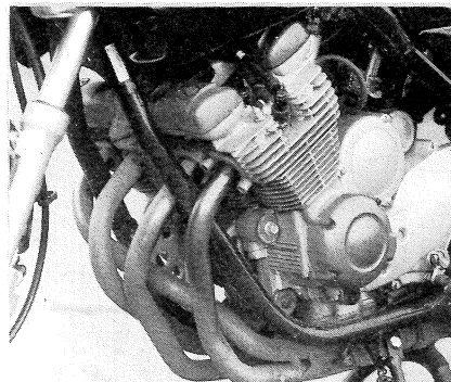
Les tubes d'échappement des cylindres, 1 et 4, et, 2 et 3, sont réunis pour un meilleur équilibrage des veines gazeuses d'échappement (photo RMT).
