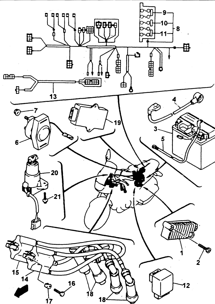
FAISCEAU PRINCIPAL ET ÉQUIPEMENTS ÉLECTRIQUES
