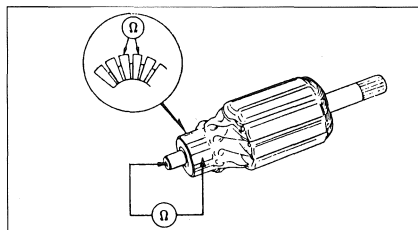
Contrôle de la continuité entre chaque lamelles et de la discontinuité entre les lamelles et l'axe.
