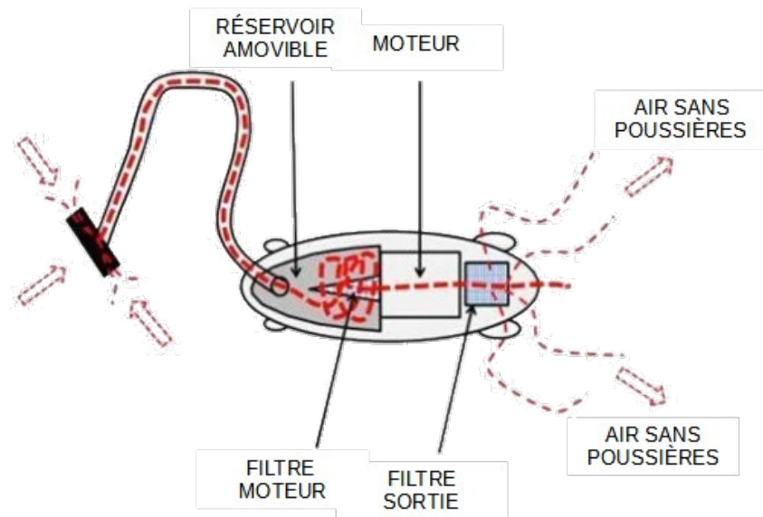
ASPIRATEUR SANS SAC
