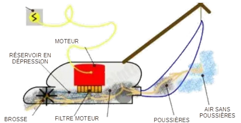
ASPIRATEUR AVEC SAC
